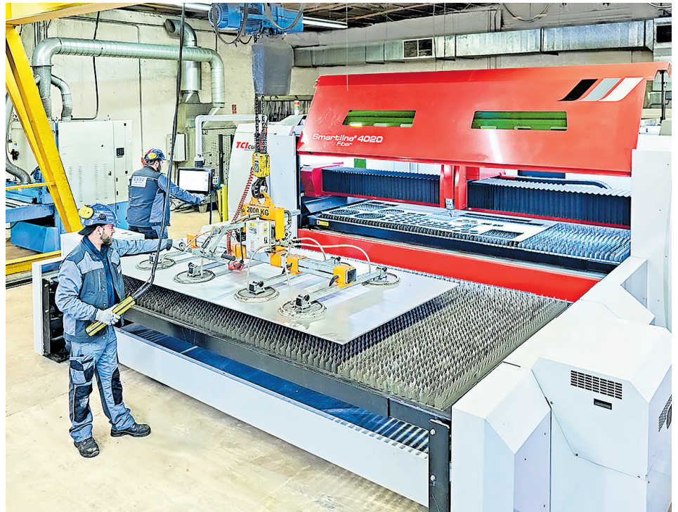
Dank der Wechseltische an den Laseranlagen wird die Maschinenauslastung optimiert. Fotos: Nikolaus Rupp
